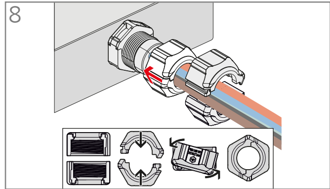
Druckschraube zusammensetzen
