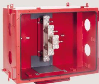
Verteilergehäuse mit Klemm- anschlüssen auf 3 Ebenen distribution box with 3 current bar terminals 11 kV
