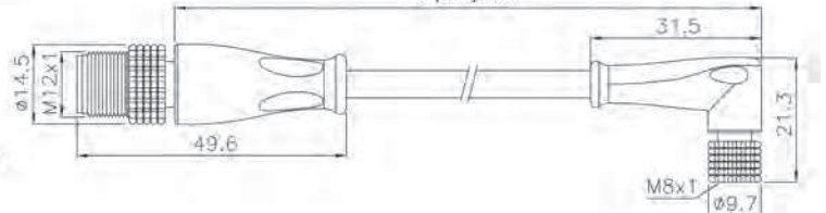
CONNETTORE M12x1 MASCHIO DIRITTO M12x1 STRAIGHT MALE CONNECTOR
