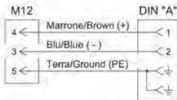
Schema elettrico Electrical diagram
