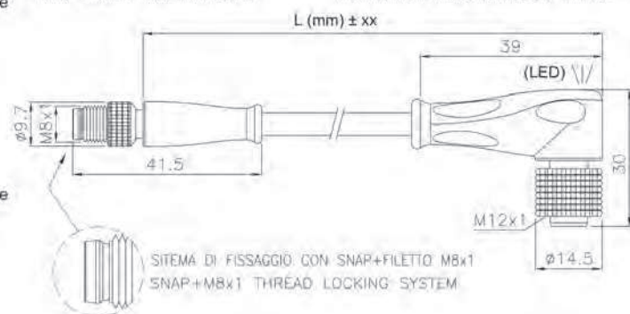
CONNETTORE M8x1 MASCHIO DIRITTO M8x1 STRAIGHT MALE CONNECTOR
