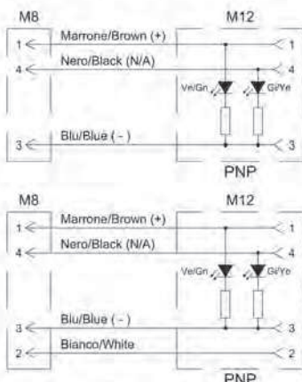
Schema elettrico Electrical diagram
